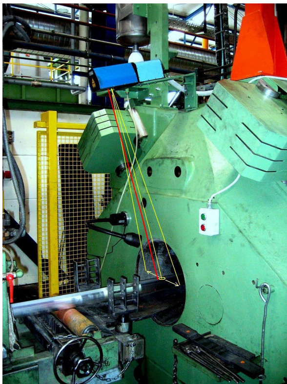
带扫描系统的红外线测温计
